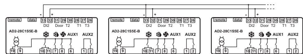
Fig.3. Conexión para la sincronización del comienzo y del término de los desescarches
